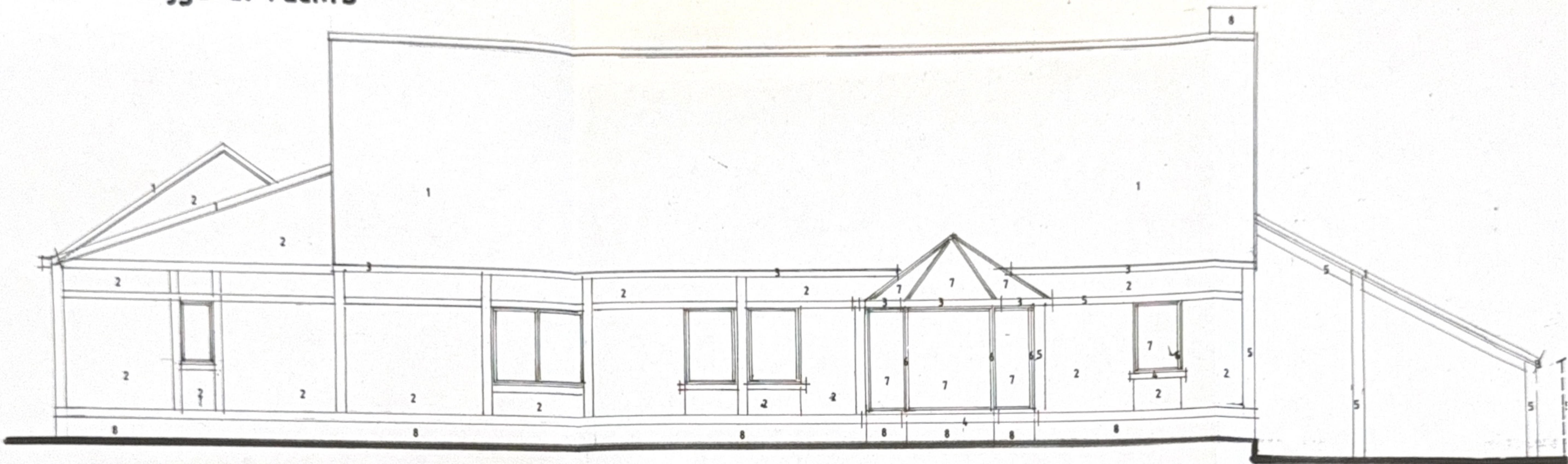
achtergevel
