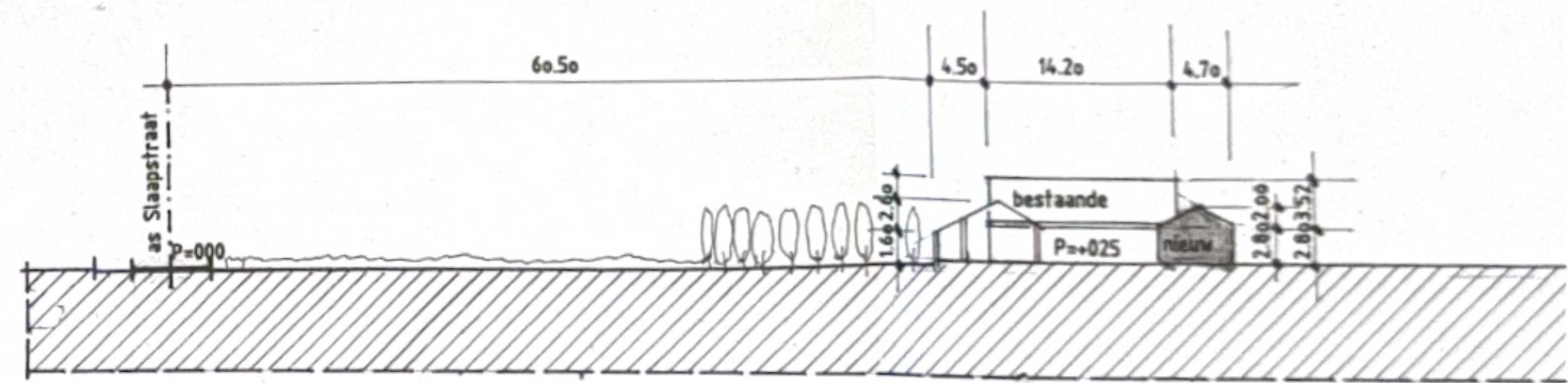
terreinprofiel 1/500°
