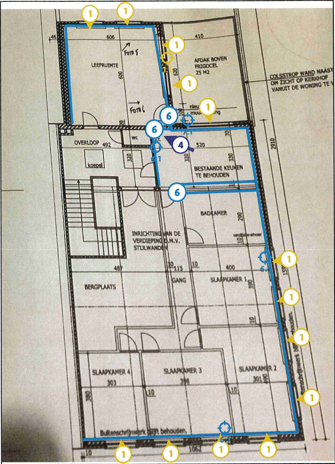
Legende van plan 1.3: Plan eerste verdieping
